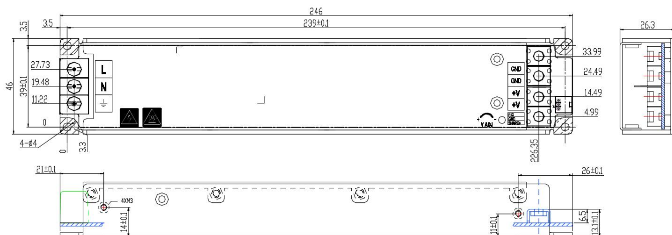
输入、输出端子定义及安装注意事项
